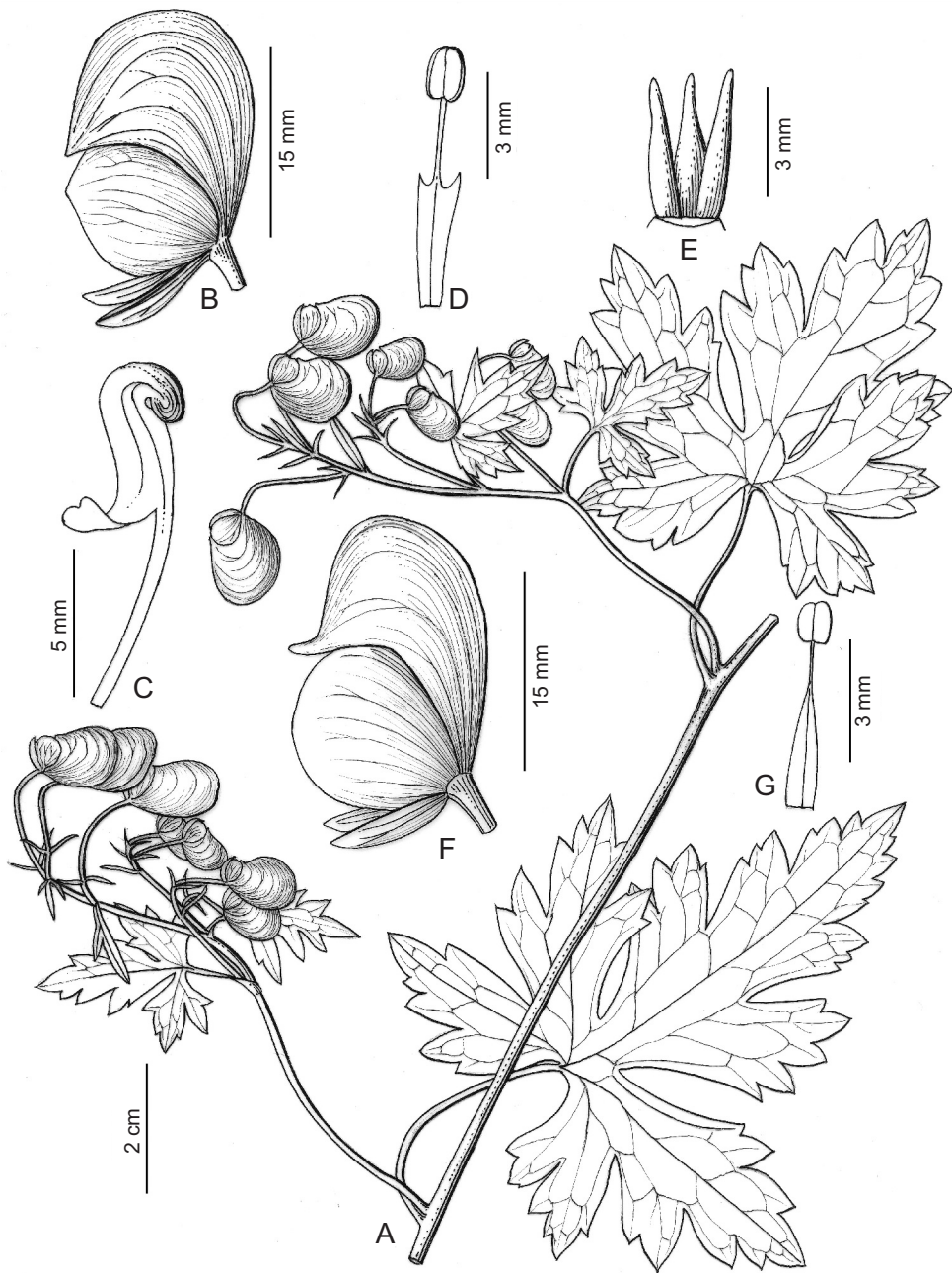
A. 开花枝一部分; B. 花; C. 花瓣; D. 雄蕊; E. 雌蕊群, 由 3 心皮组成; F. 花; G. 雄蕊。 A. Part of flowering branch; B. Flower; C. Petal; D. Stamen; E. Gynoecium, consisting of three carpels (from holotype); F. Flower; G. Stamen. (K. M. Feng 6957)
