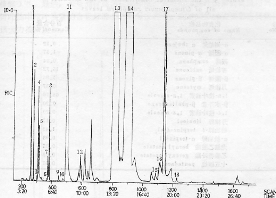
图2 咸丰产川桂叶精油总离子流图
