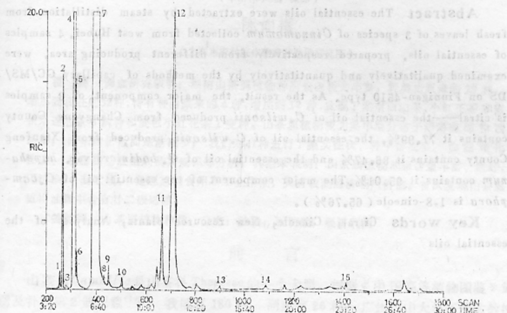
图4 樟叶精油总离子流图
